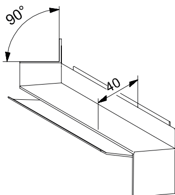
Verbinder für Außenecke, 90 Grad
