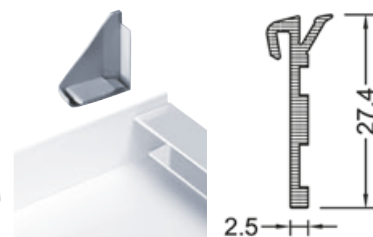
Dichtstück und Anschlussdichtung UD 40-25
