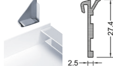
Dichtstück und Anschlussdichtung UD 40-25
