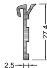
Dichtstück und Anschlussdichtung UD 40-25
