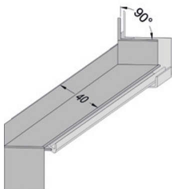
Verbinder für Außenecke, 90 Grad
