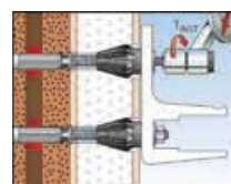
10 Anbauteil befestigen, angegebenes Drehmoment aufbringen.
