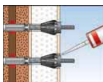
9 Ringspalt zu Putz mit fischer Dichtkleber verfüllen.
