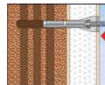
5 Siebhülse einschieben.
