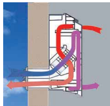
Funktionsschema
