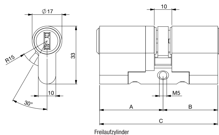
Zahnritzelzylinder
