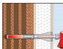
6 Mörtel FIS V einfüllen.
