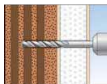
1 Bohrloch herstellen.
