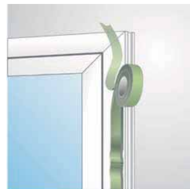
Stumpfstoß bei der Fenstermontage
